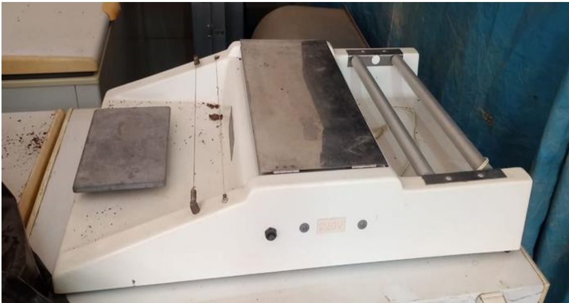
01 - Embaladora/filmadora, fabricante J. C. Brey
